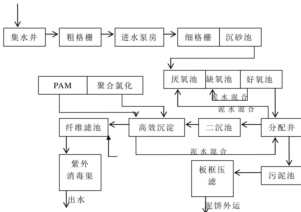
澄西污水处理厂工艺流程图
